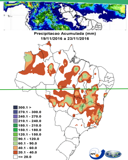
Figura 1 Fontes de dados: CPTEC/INPE INMET FUNCEME/CE AESA/IB EMPAR/RN ITEP/LAMEPE/PE DHME/PI CMR/SE SEMAR/DH/AL COMET/RJ SEMAR/BA-CEMIG/SIMO/MG-SEAG/ES-SIME/PA/PR-CLIM/ER/SC-AC/IS/P A 12 Noite/AQUA UMD Tarde )
