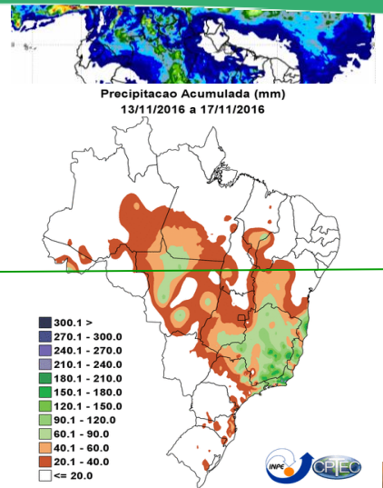
Figura 1 Fontes de dados: CPTEC/INPE INMET FUNCEME/CE AESA/IB EMPAR/RN ITEP/LAMEPE/PE DHME/PI CMRH/SE SEMAR/DH/AL COMET/RJ SEMAR/BA-CEMIG/SIMGE/MG-SEAG/ES-SIMEPAR/PR-CLIMERRH/SC-IAC/SP 1 00:00:00 A 2016-11-21 23:59:59 (A 12 Noite/AQUA UMD Tarde)
