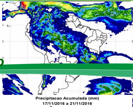
Figura 1 Fontes de dados: CPTEC/INPE INMET FUNCEME/CE AESA/IB EMPAR/RN ITEP/LAMEPE/PE DHME/PI CMR/SE SEMAR/DH/AL COMET/RJ SEMAR/BA-CEMIG/SIMO/MG-SEAG/ES-SIME/PA/PR-CLIM/ER/SC-AC/IS/P A 12 Noite/AQUA UMD Tarde )
