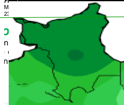
Instituto Nacional de Meteorologia - INMET Precipitação Acumulada nos últimos 5 dias Mapa do dia 20/09/2016
