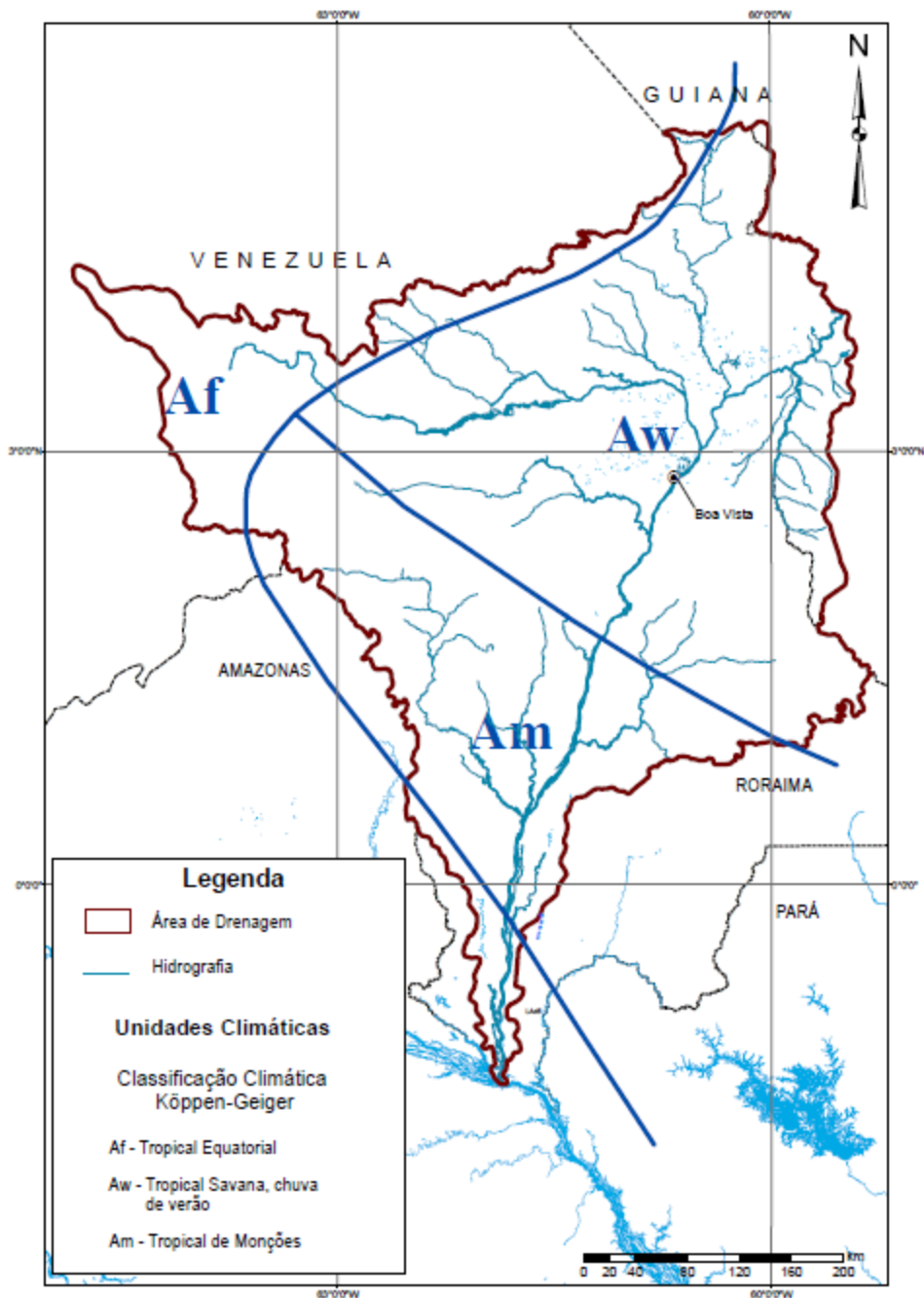
Figura 17. Classificação Climática de Köppen e sua Distribuição Espacial em Roraima
