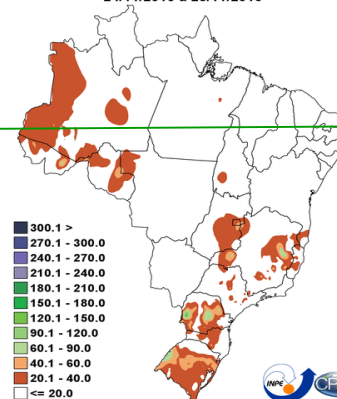
Fontes de dados: CPTEC/INPE INMET FUNCEME/CE AESA/PB EMPARN/RN ITEP/LAMEPE/PE DHME/PI CMRH/SE SEMARH/DHNA/AL COMET/RJ SEMARH/BA-CEMIG/SIMIG/MS-SEAG/ES-SIMEPAR/PR-CLIME/RHCC/AC/SP
