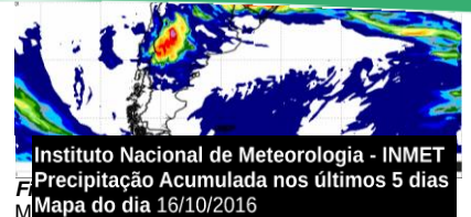
Instituto Nacional de Meteorologia - INMET Precipitação Acumulada nos últimos 5 dias Mapa do dia 16/10/2016
