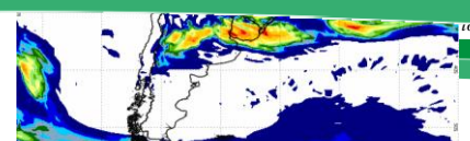
Instituto Nacional de Meteorologia - INMET Precipitação Acumulada nos últimos 5 dias Mapa do dia 17/10/2016
