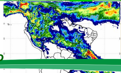
Figura 1 Fontes de dados: CPTEC/INPE INMET FUNCEME/CE AESA/IB EMPAR/RN ITEP/LAMEPE/PE DHME/PI CMRH/SE SEMAR/DH/AL COMET/RJ SEMAR/BA-CEMIG/SIMGE/MG-SEAG/ES-SIMEPAR/PR-CLIMERRH/SC-IAC/SP 4 focos de 2016-11-1 a 2016-11-19 no RR mandatada em 11/11/2016
