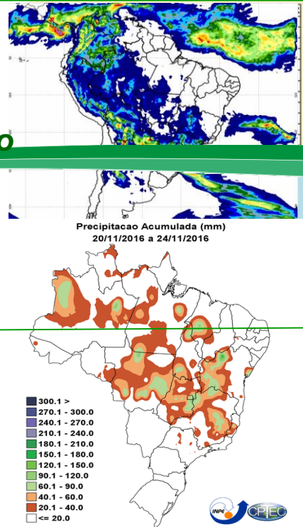
Figura 1 19 focos de 2016-11-1 a 2016-11-28 no RR mandado RR
