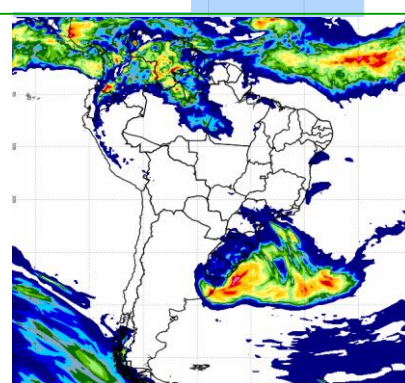
Figura 2- Modelo COSMO (7x7km) - INMET. Modelo de precipitação acumulada para o dia 7/9/2016
