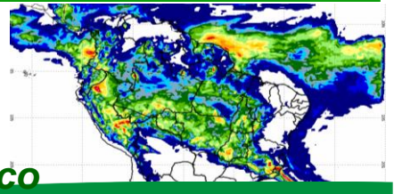
Fontes de dados: CPTEC/INPE INMET FUNCEME/CE AESA/IB EMPARN/RN ITEP/LAME/PE/PE DIME/PI CMR/SE SEMARH/DH/AL COMET/RJ SEMARH/BA-CEMIG/SIMGE/MG-SEAG/ES-SIMEPAR/PR-CLIMERH/SC-IAC/SP Figura 1
