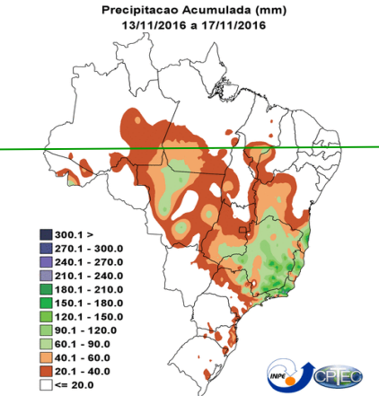
Figura 1 Fontes de dados: CPTEC/INPE INMET FUNCEME/CE AESA/IB EMPAR/RN ITEP/LAMEPE/PE DHME/PI CMRH/SE SEMAR/DH/AL COMET/RJ SEMAR/BA-CEMIG/SIMGE/MG-SEAG/ES-SIMEPAR/PR-CLIMERRH/SC-IAC/SP 4 focos de 2016-11-1 a 2016-11-19 no RR mandatada em 11/11/2016
