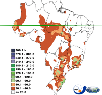
Fontes de dados: CPTEC/INPE INMET FUNCEME/CE AESA/PB EMPAR/NRN IPT/LAME/PE/DHME/RJ CMR/ISE SEMARH/DHVAL/COMETR/JR SEMARH/BA-CEMIG/SIMGE/MS-SEAO/ES-SIMEPAR/PR-CLIMRHS-AC/SP
