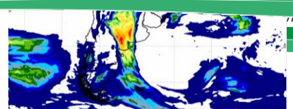
Figura 2- Modelo COSMO (7x7km) - INMET. Modelo de precipitação acumulada para o dia 5/10/2016
