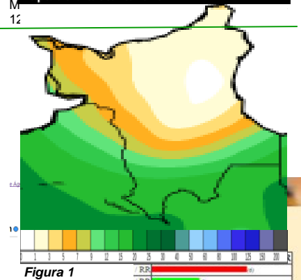
Instituto Nacional de Meteorologia - INMET Precipitação Acumulada nos últimos 5 dias Mapa do dia 09/10/2016
