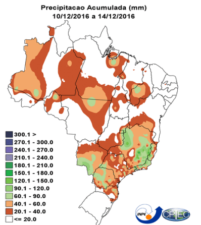
Fontes de dados: CPTEC/INPE INMET FUNCEME/CE AESA/IB EMPARN/RN ITEP/LAME/PE/PE DIME/PI CMR/SE SEMARH/DH/AL COMET/RJ SEMARH/BA-CEMIG/SIMGE/MG-SEAG/ES-SIMEPAR/PR-CLIMERH/SC-IAC/SP Figura 1
