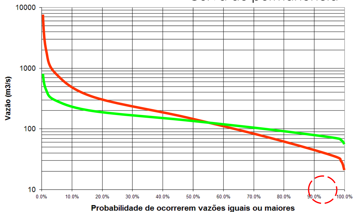
Curva de permanência
