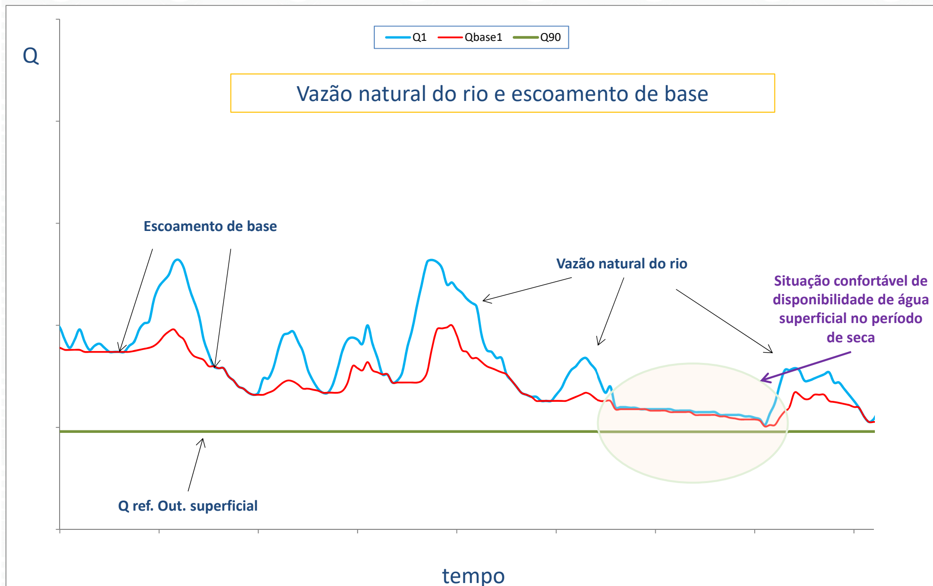
Hidrograma com separação de escoamentos (ANA, 2013)
