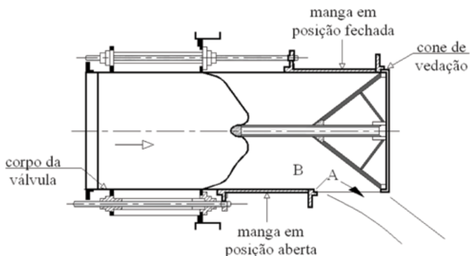
Figura 7 – Válvula de jato oco
