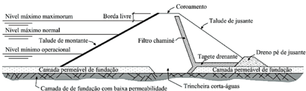
Figura 2 - Seção transversal de uma barragem de terra homogênea
