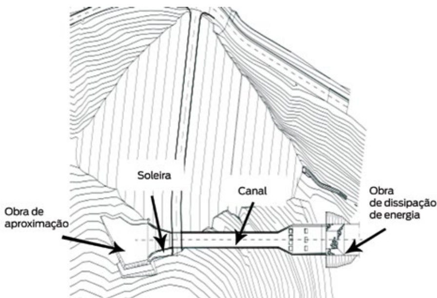
Figura 4 – Planta esquemática de vertedouro em canal de encosta e bacia de dissipação de energia
