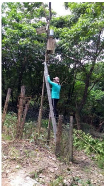
Figura 6 - Atualização modem GOES – Porto Calvo – Julho/2019
